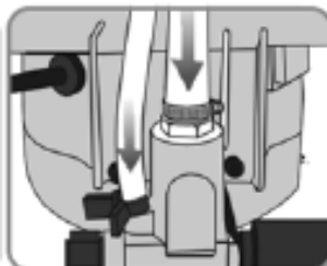
9 - RECONECTE OS TUBOS E PRENDA COM ABRAÇADEIRAS
