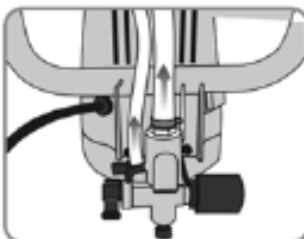
2 - VIRE A UNIDADE E SOLTE OS GRAMPOS DE AMBOS OS TUBOS E DESCONECTE OS TUBOS DO CORPO DA BOMBA
