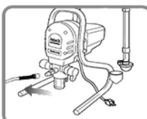
15 - PARA SABER SE A BOMBA E OS TUBOS ESTÃO PREPARADOS PARA O USO, O MOTOR DEVE PARAR. CASO NÃO PARE, REPITA OS PASSOS DE PREPARAÇÃO 15
